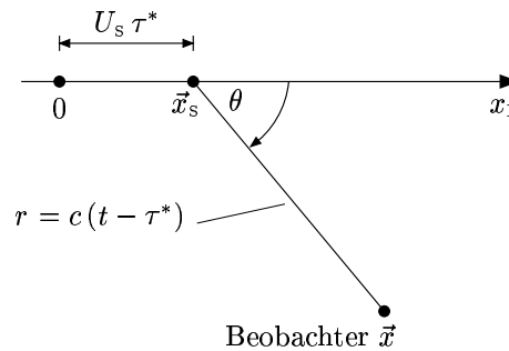
Abbildung 9.4: Zur Definition des Winkels \theta zwischen Beobachtungs- und Bewegungsrichtung.
