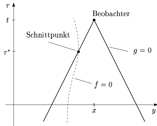
Abbildung 10.5: Betrachtung der Mengen f = 0 und g = 0 bei einer Raumdimension: y \in \mathbb{R} .
