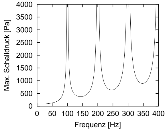
Abbildung 3.9: Maximale Druckamplitude als Funktion der Frequenz (Rohrlänge L = 1.7 m und Auslenkung \varepsilon = 1 mm)
