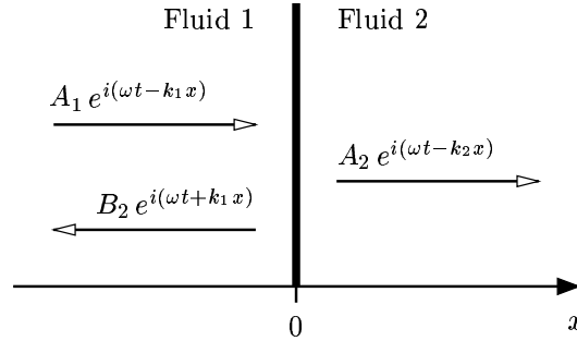
Abbildung 3.13: Einfallende ( A_1 ), reflektierte ( B_1 ) und transmittierte ( A_2 ) Welle an der Mediengrenze bei x = 0 .
